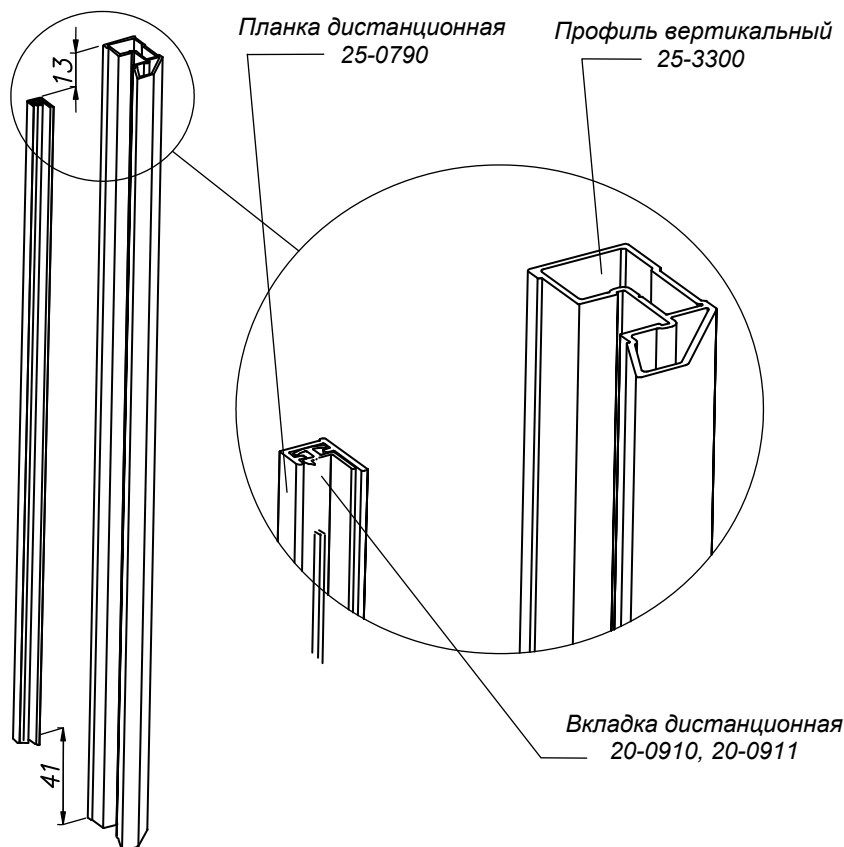
Рис. 8 Монтаж вертикально профиля Szařir перед забивкой его на стекло 4-4.6 мм
