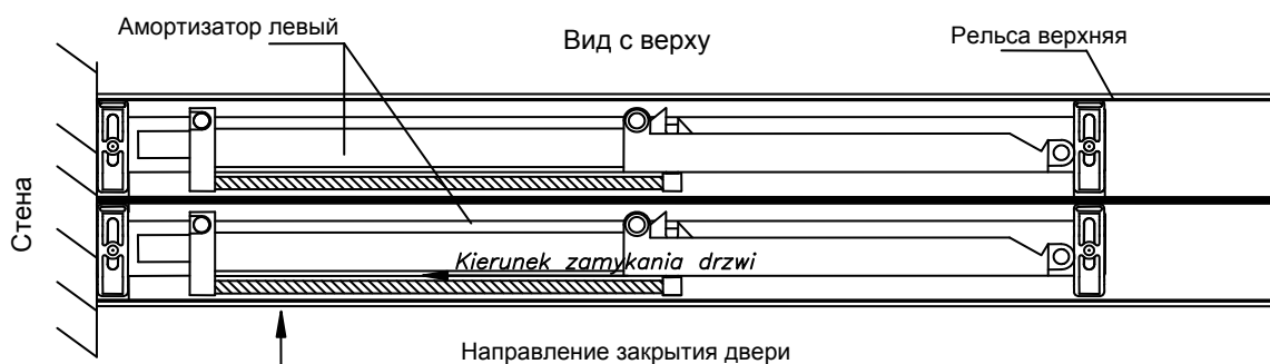
Рис.27 Монтаж газового доводчика в верхнюю рельсу
